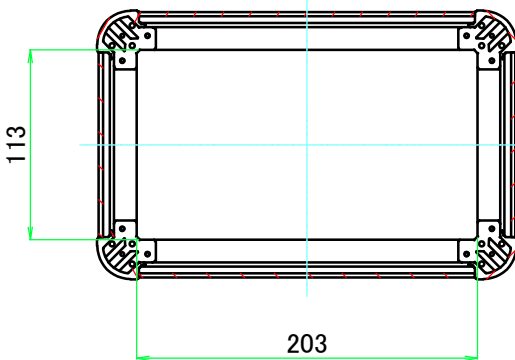
C-C ( 1 : 4.5 )
